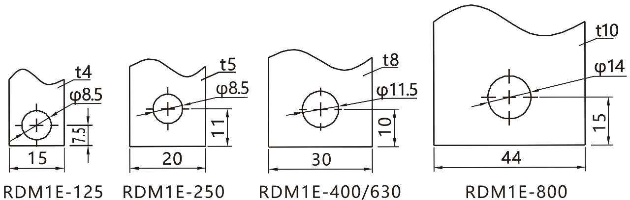
图13 RDM1E系列推荐预制铜排尺寸
