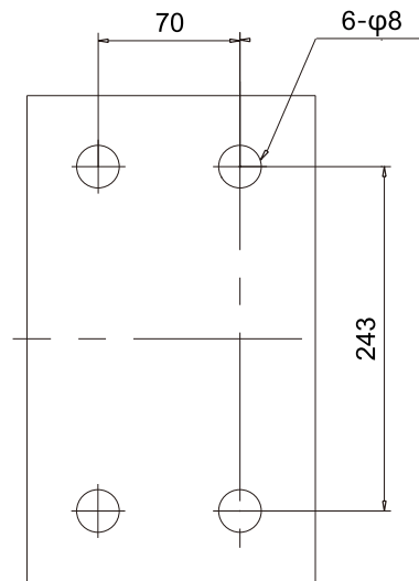
RDM1E-1250安装底板开孔
