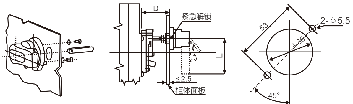
“F”型方形手柄外形柜门开孔尺寸(开孔中心离铰链距离不小于100mm)
