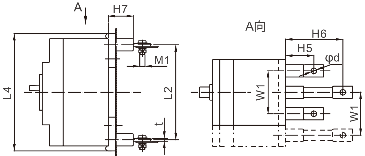
图4 RDM1E-400、630、800固定式板后接线
