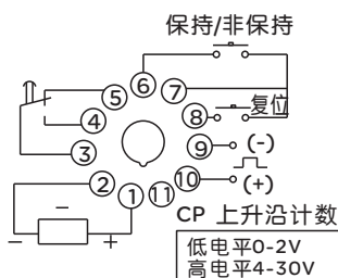
图4 RDJ1-48-11直流脉冲计数接线图
