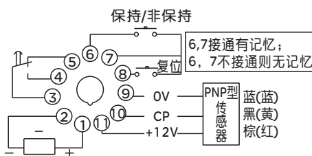
图3 RDJ1-48-11传感器计数接线图
