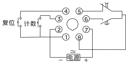
图1 RDJ1-48-8接点计数接线图
