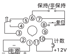
图2 RDJ1-48-11接点计数接线图
