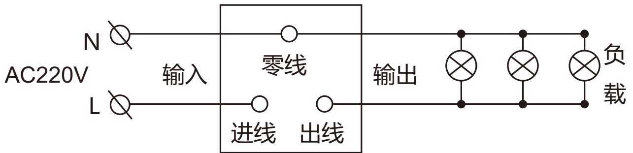
图1 GUK-81、-82、-83、-84接线图
