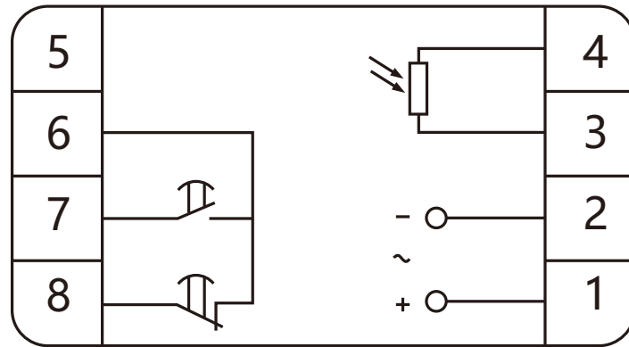
图2 GUK-82(KG-2)接线图
