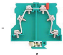
(5) JF5试验型接线座(S3)
