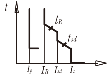
电子式脱扣器保护特性曲线
