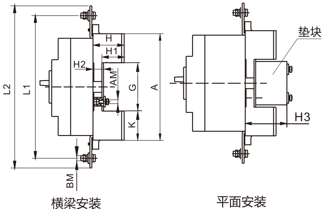
图7 插入式板前接线(单位:mm)
