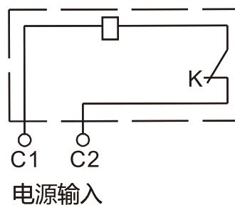
图12 AC50Hz 230V、400V接线图
