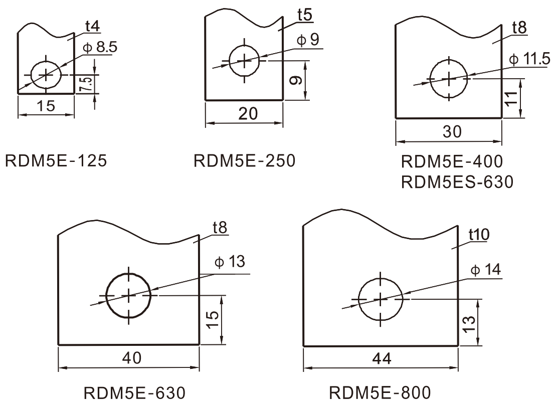
图14 RDM5E系列推荐预制铜排尺寸
