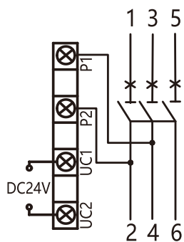
图11 DC24V接线图
