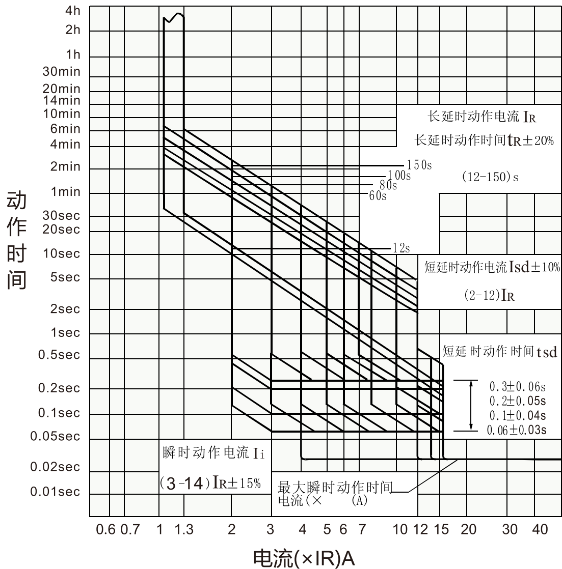
图1 RDM5E-125-800型脱扣特性曲线
