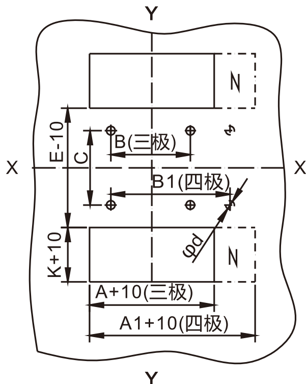
图10 插入式板厚接线安装板开孔尺寸(单位:mm)
