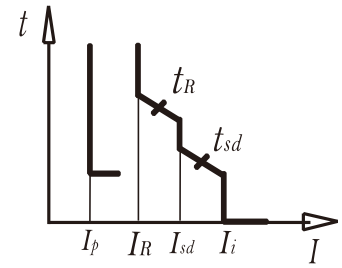
电子式脱扣器保护特性曲线
