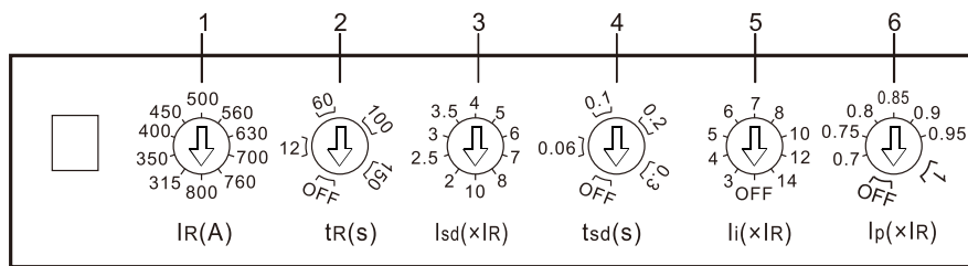
RDM5E-800, I_n=800A 电子式脱扣器
