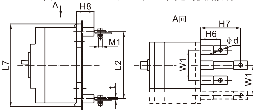
图4 RDM5E-400、630、800固定式板后接线
