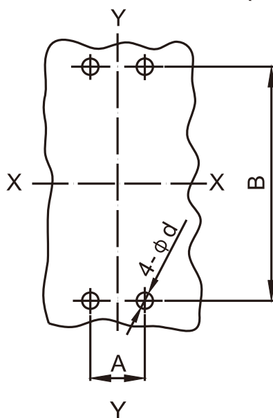
图5 板前接线安装板开孔尺寸
