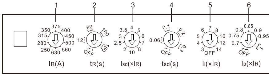
RDM5E-630, I_n=630A 电子式脱扣器
