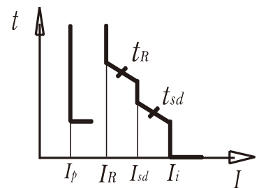
电子式脱扣器保护特性曲线
