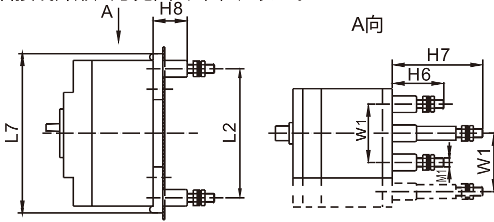
图3 RDM5E-100、125、250固定式板后接线
