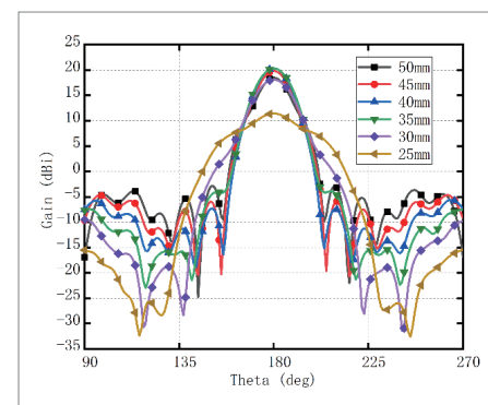
E 面方向图
