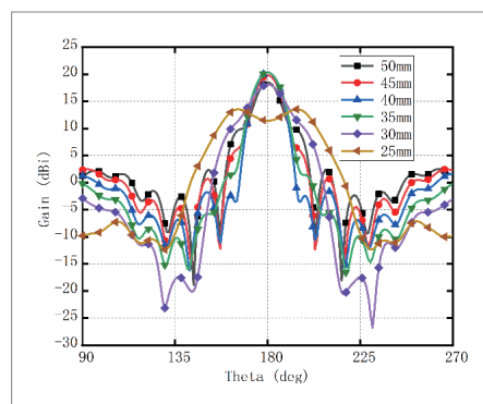
H 面方向图
