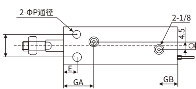
共同尺寸表
