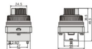
选择型旋钮
