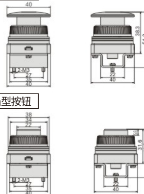
大圆型按钮
