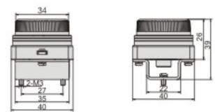
平型按钮
