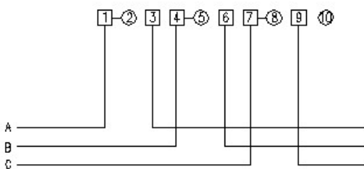
三相三线直接接入式
