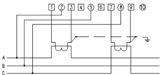
三相三线电流互感式接入式接线图
