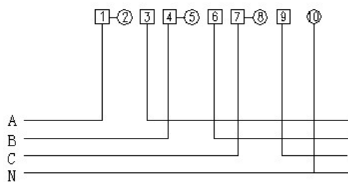
三相四线直接接入式
