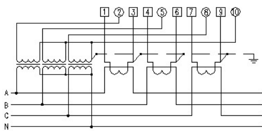
三相四线经电流电压互感器接入式
