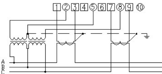
三相三线电压、电流互感式接入式接线图
