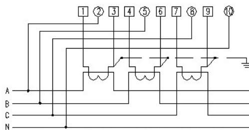
三相四线经电流互感器接入式
