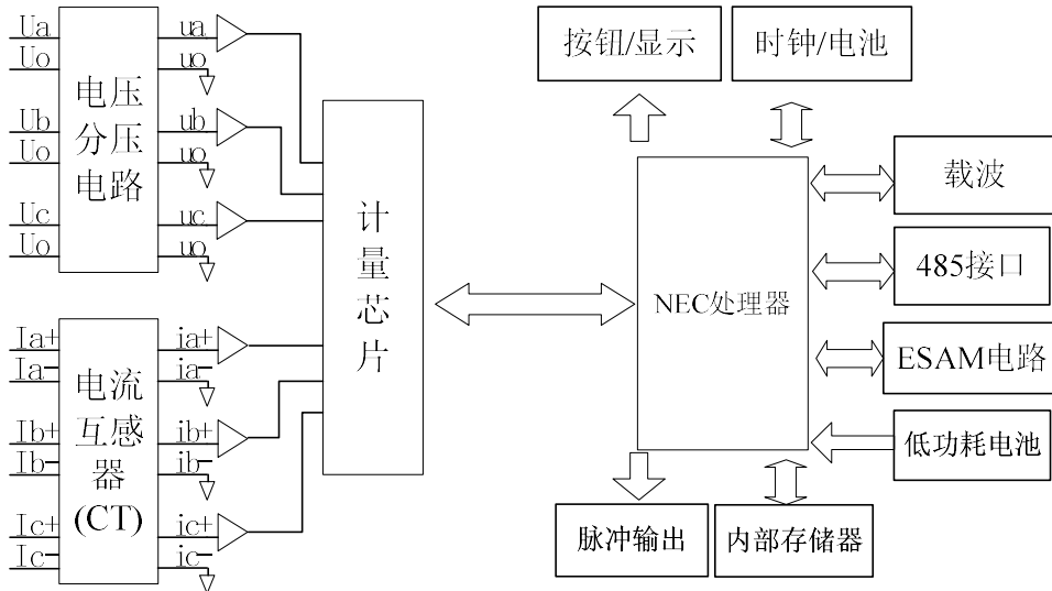
图 1：电能表基本工作原理
